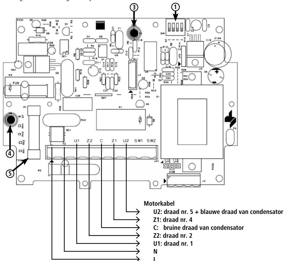
Afbeelding 7: Schema hoofdprintplaat
