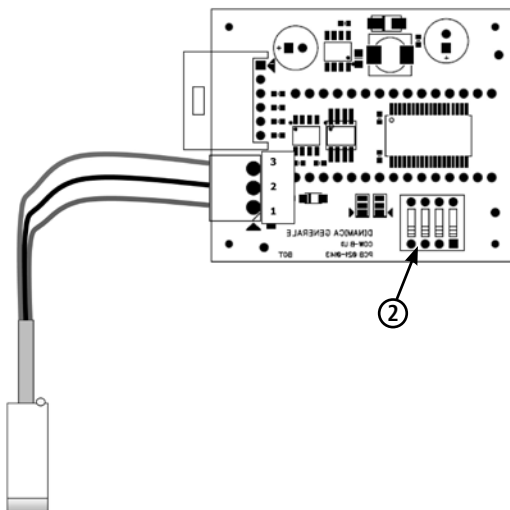
Kuva 8: Päohjauskortin kaavio + anturin liitäntä
