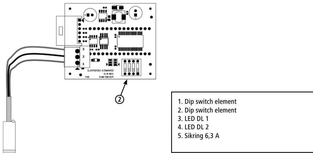
Illustration 8: Skema displaykort + tilslutning sensor
