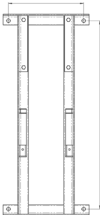
Ilustracja 3: Schemat otworów
