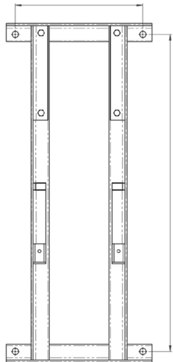
Afbeelding 3: Boorsjabloon
