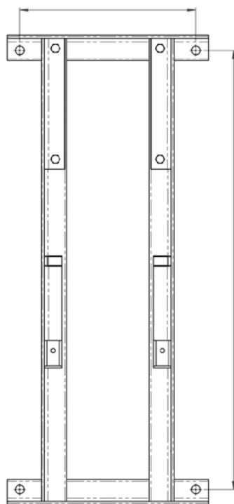
Bild 3: Hålbild
