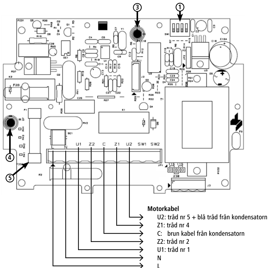
Bild 7: Schema huvudstyrkort
