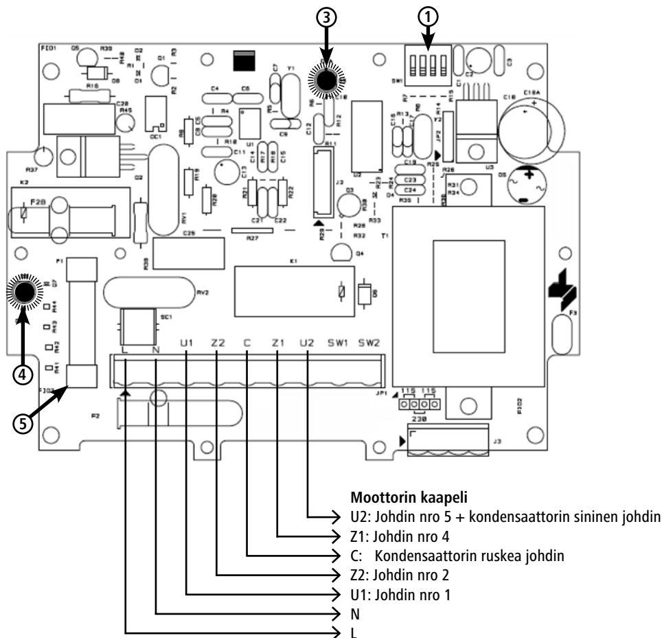
Kuva 7: Pääohjauskortin kaavio
