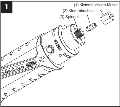
1 (1) Collet Nut | Dado della bussola di fissaggio | Spantangmoer | Bilezik Somunu | Ecrou de serrage (2) Collet | Bussola di fissaggio | Spantang | Bilezik | Douille de serrage (3) Spindle | Mandrino | As | Mil | Broche
