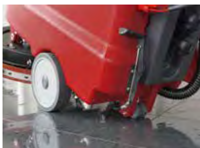
Über das Stützrad kann die Maschine einfach transportiert oder Bürsten schonend abgestellt werden.
