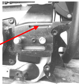
Ölzufuhr- öffnung
