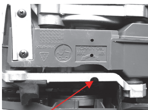
Einstellschraube
